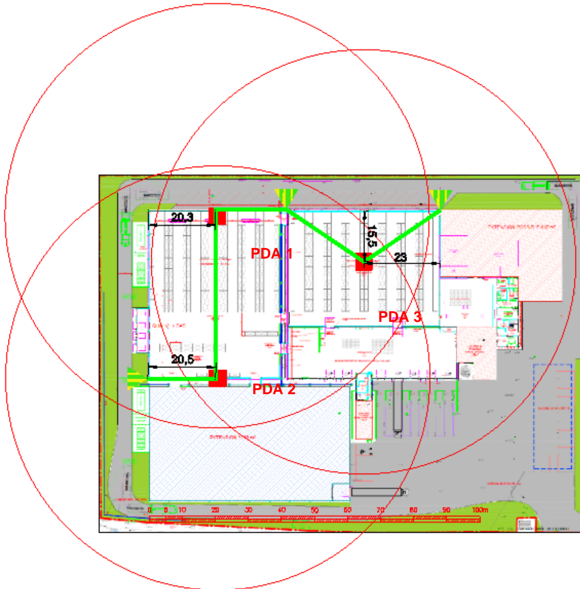
Figure 12 : Implantation des paratonnerres
